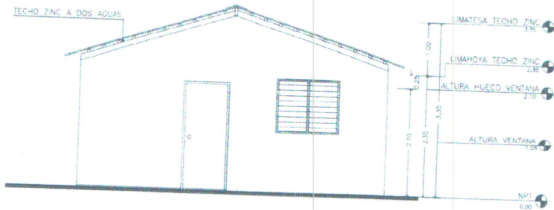
Elevación Posterior
