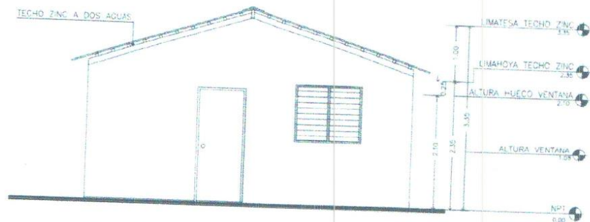
Elevación Posterior
