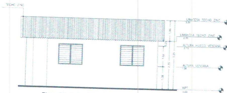
Elevación Lateral Izquierda
