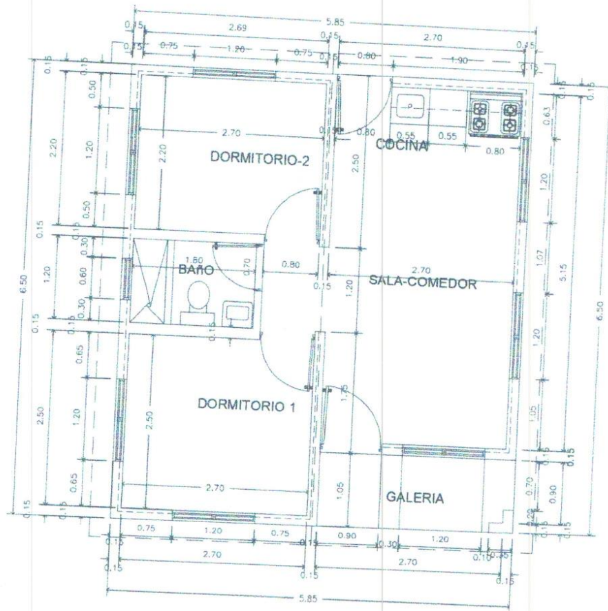
Planta Arquitectónica Dimensionada Vivienda Tipo A-1 de Block y Zinc 38.00 m2 ESC.1:50
